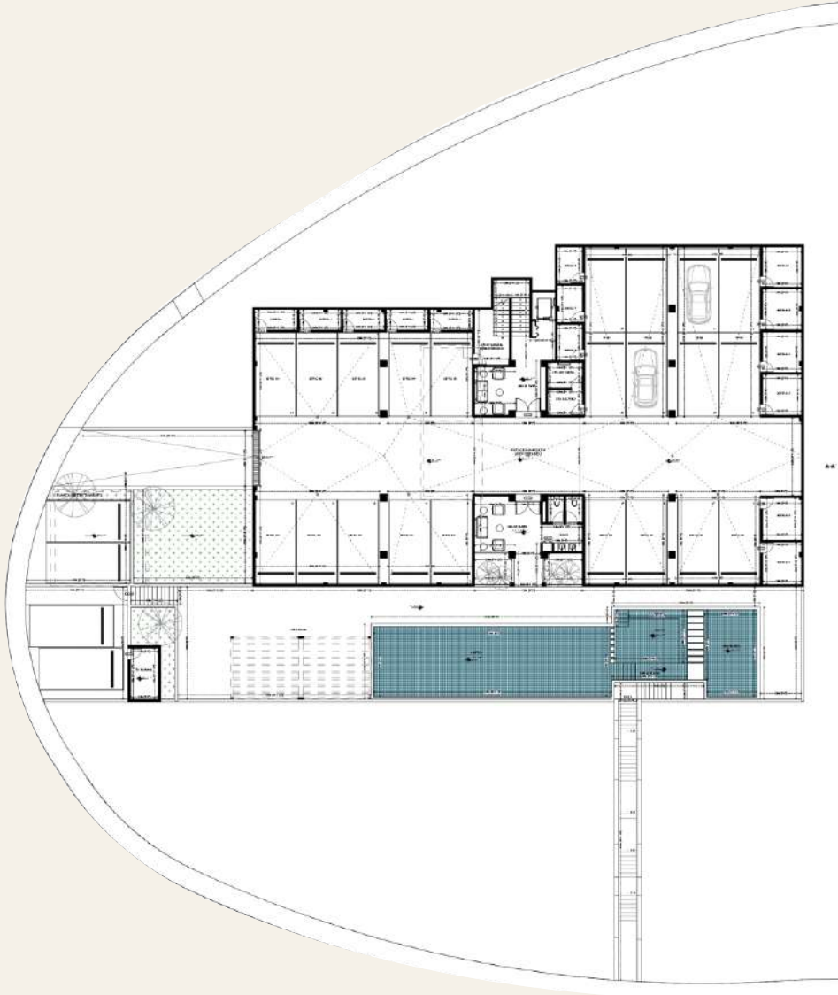
Architectural plan of parking Planta arquitectónica de estacionamiento
